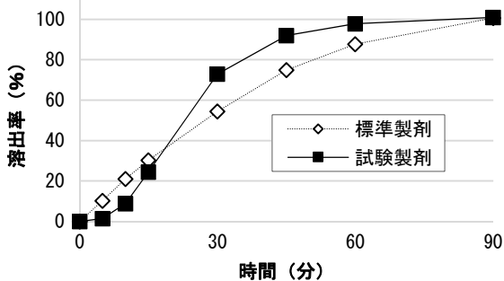
溶出試験第2液、100回転
