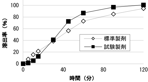
溶出試験第2液、50回転
